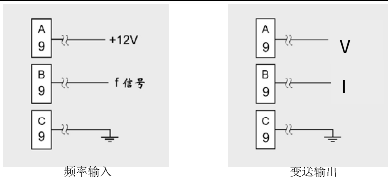
图 2-2-5 频率输入、变送输出接线图
