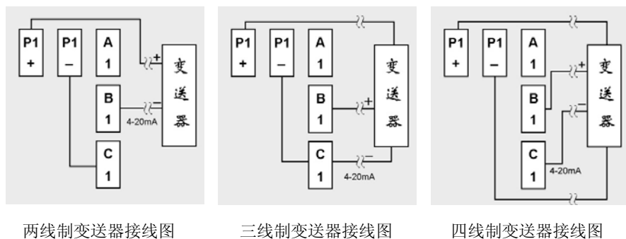
图 2-2-6 带馈电变送器接线图
