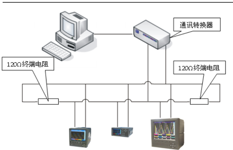
图 2-2-8 485 通讯联网示意图
