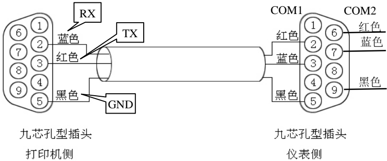
图 2-2-7-B 打印机与仪表间的 RS-232C 通讯线
