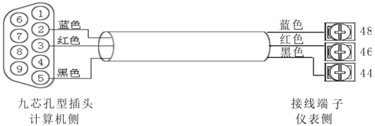
图 2-2-6-A 计算机与仪表间的 RS-232C 通讯线
