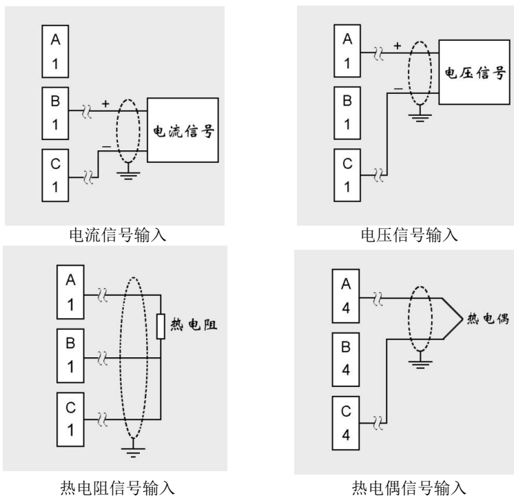
图 2-2-4 模拟量输入信号接线图
