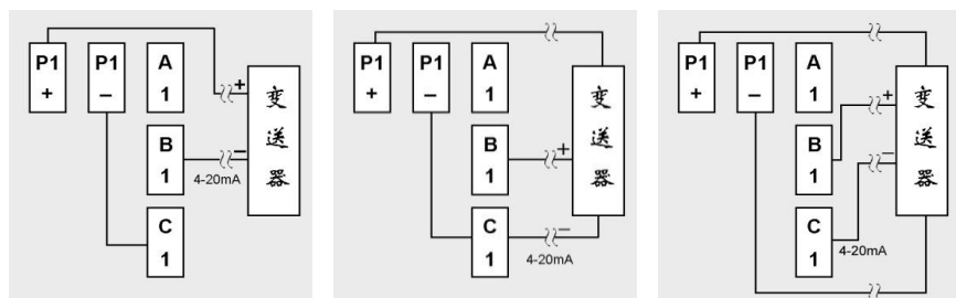
图 2-2-4 模拟量输入信号接线图
