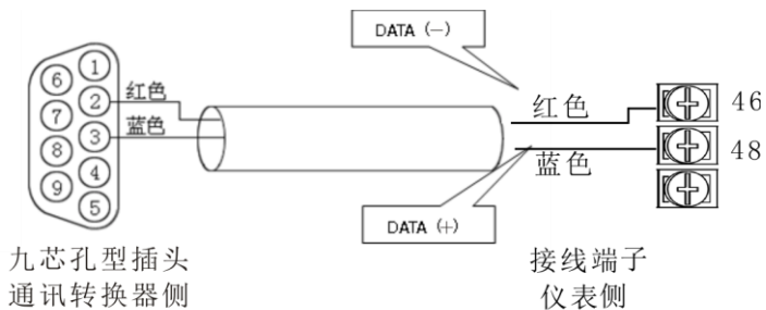
图 2-2-8 485 通讯联网示意图
