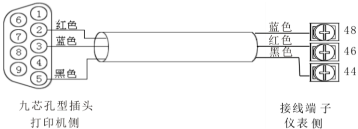
图 2-2-6-B 打印机与仪表间的 RS-232C 通讯线
