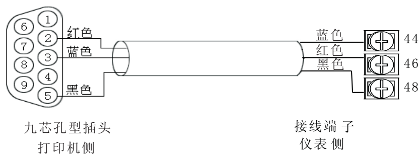
打印机与仪表间的RS-232C通讯线
