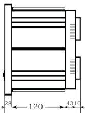
侧视图
