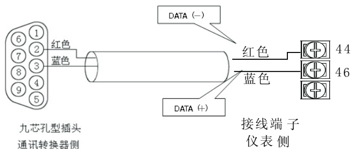
通讯转换器与仪表间的485通讯线
