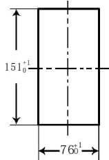
开孔图
